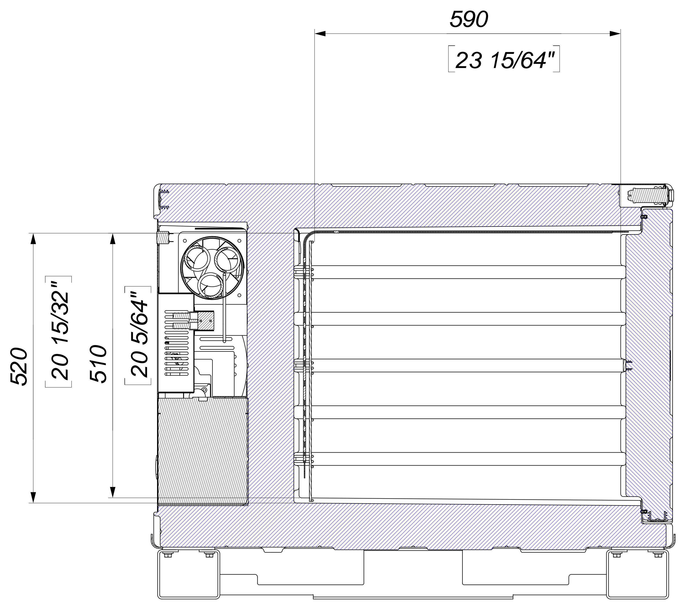
Sezione E-E SCALE 1 : 3.50
