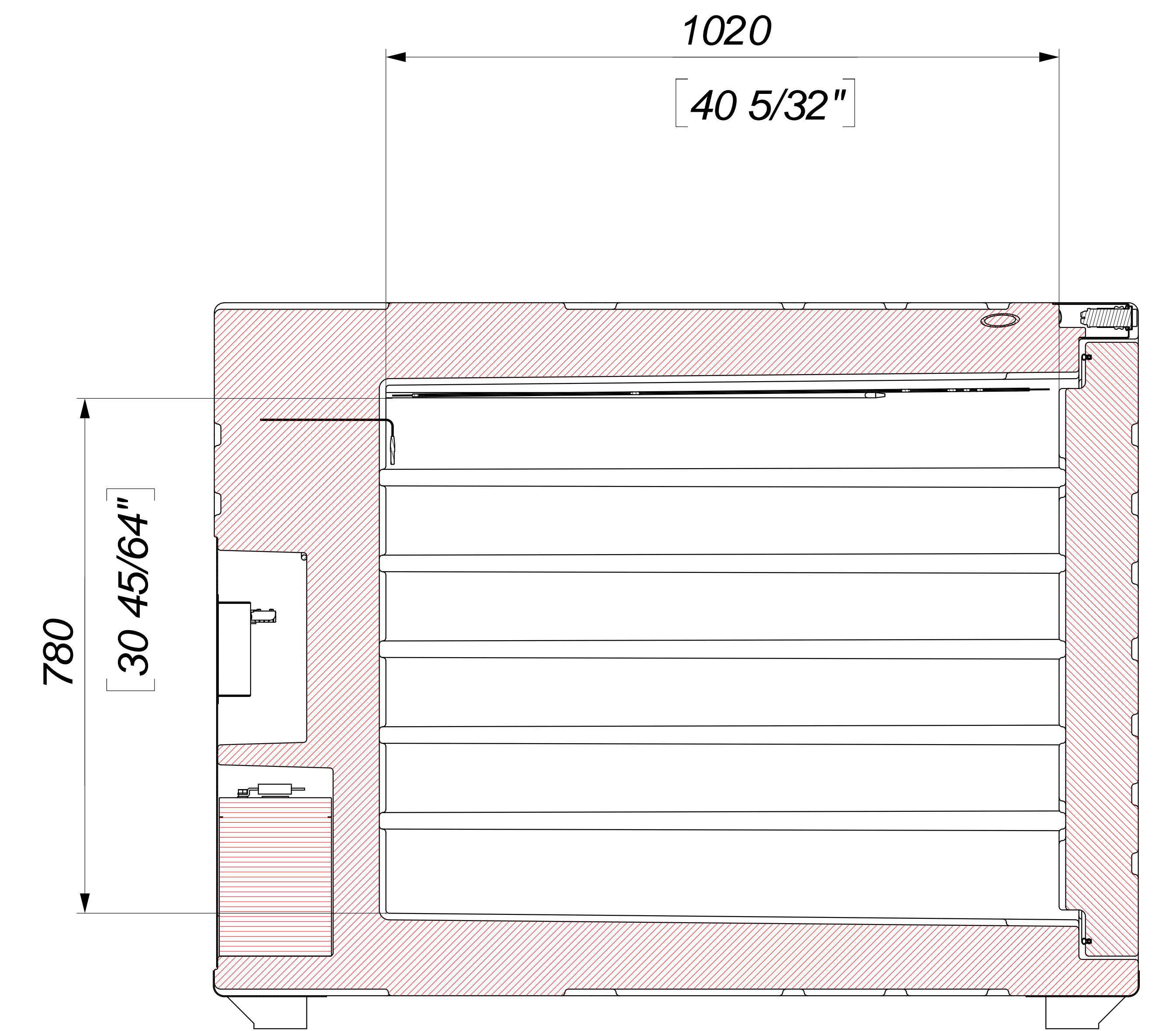
Sezione E-E SCALE 1:5
