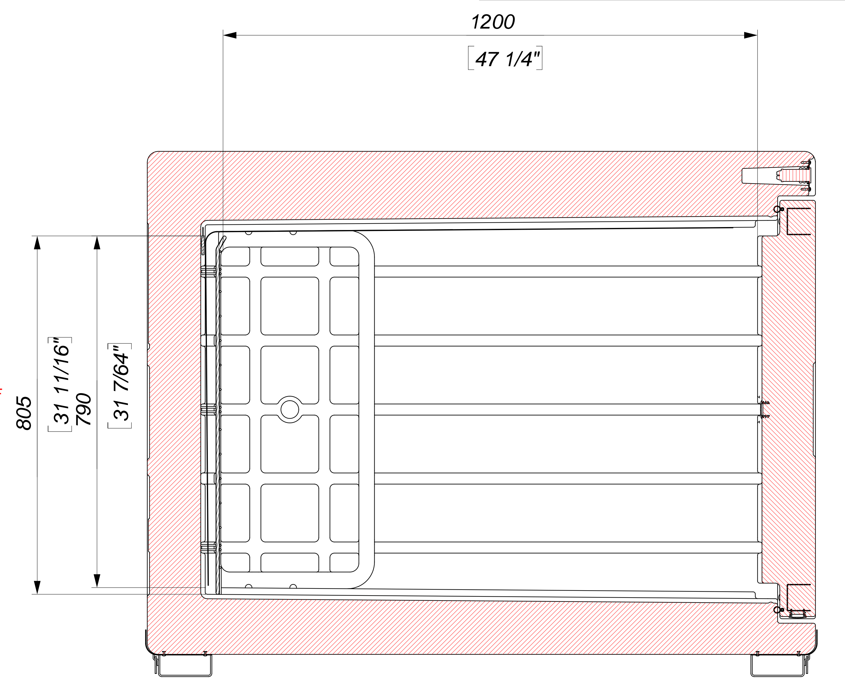
Sezione E-E SCALE 1 : 5
