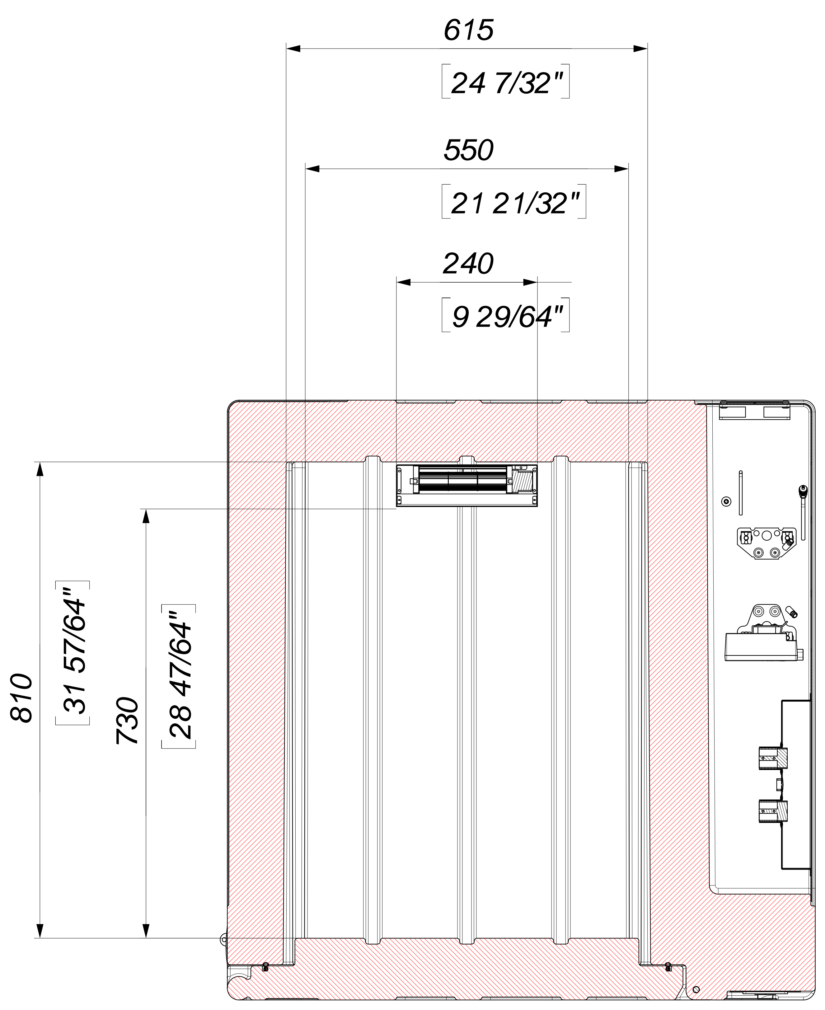
Sezione F-F SCALE 1 : 4
