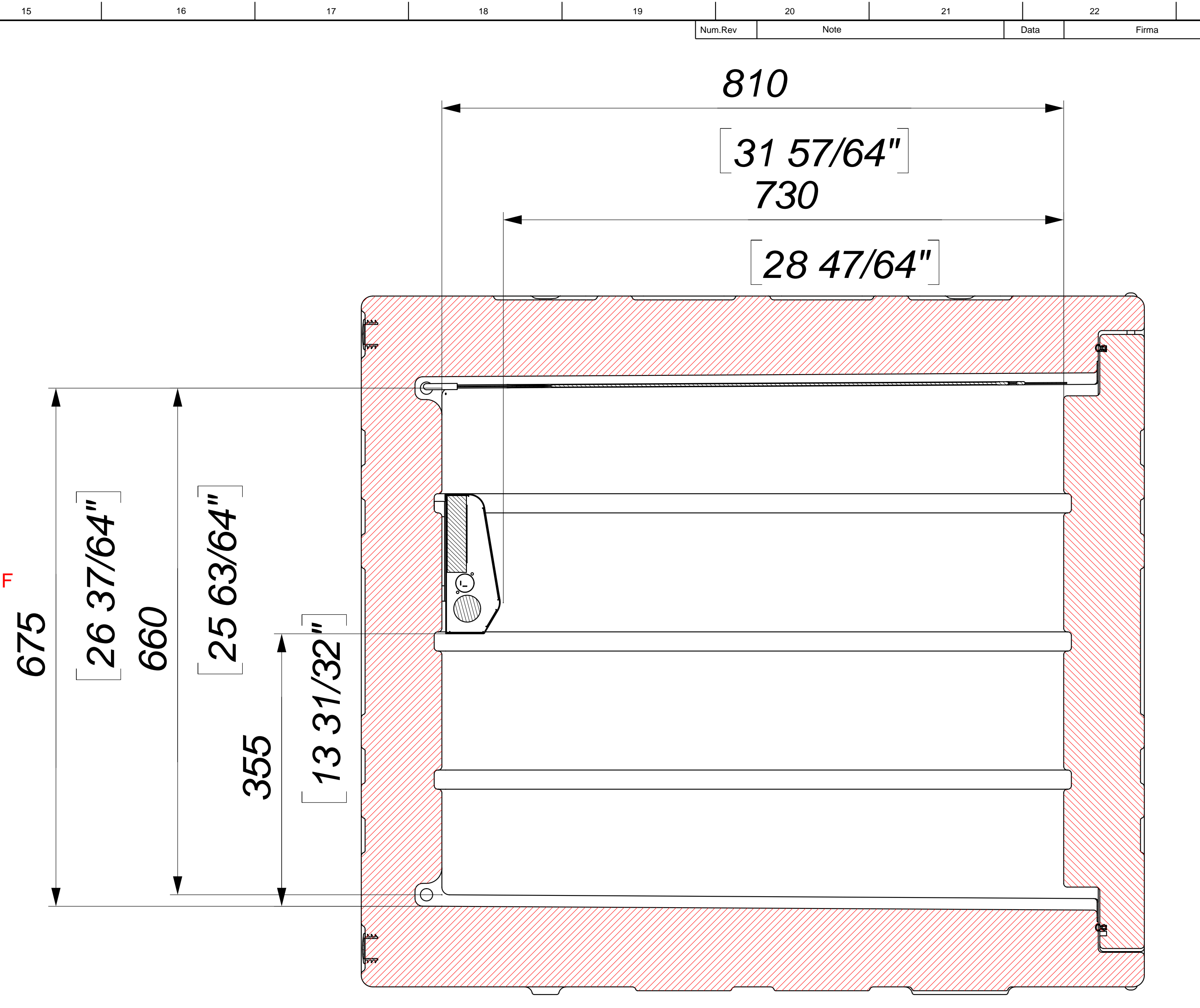
Sezione E-E SCALE 1 : 4
