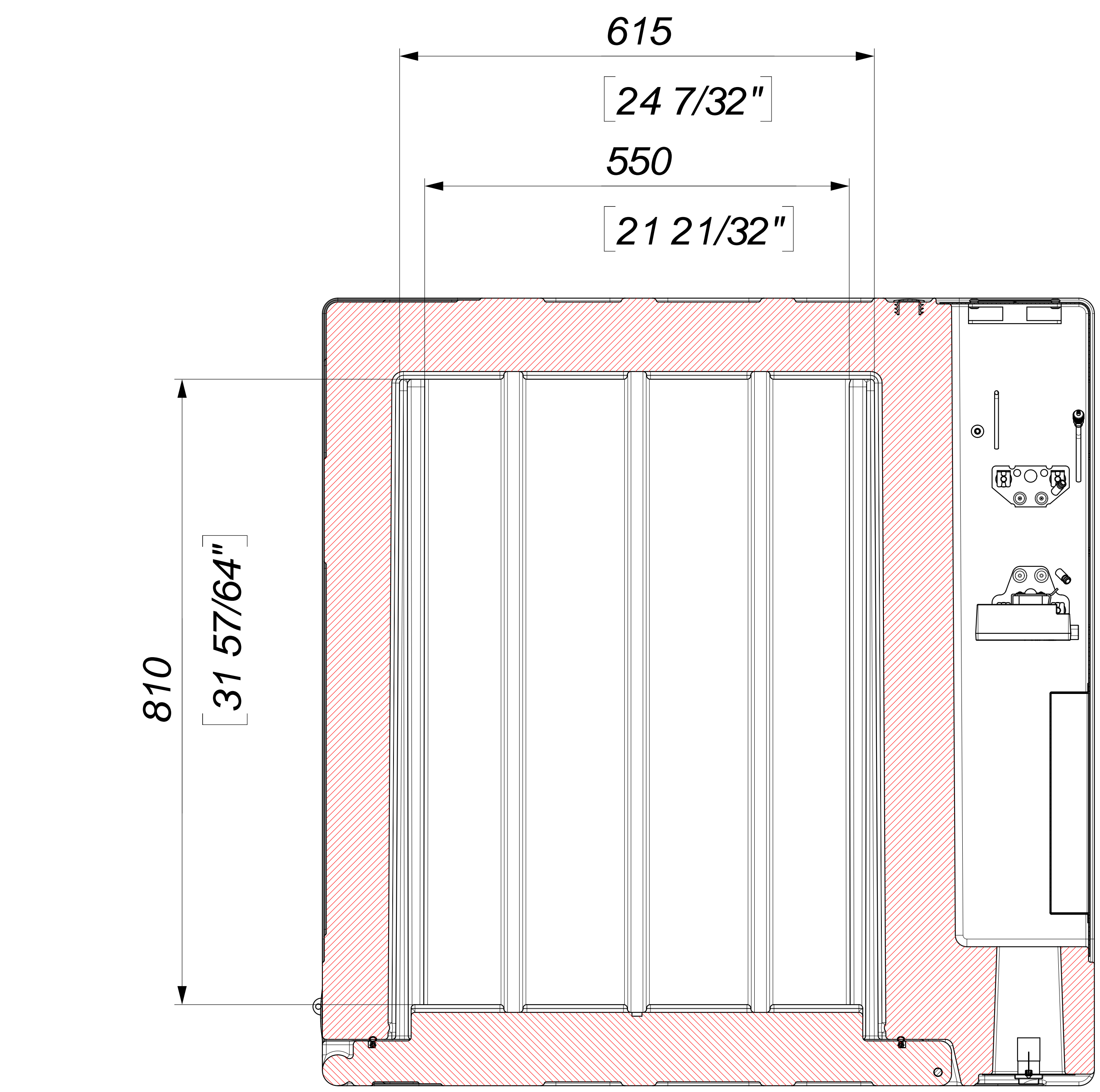
Sezione F-F SCALE 1 : 4
