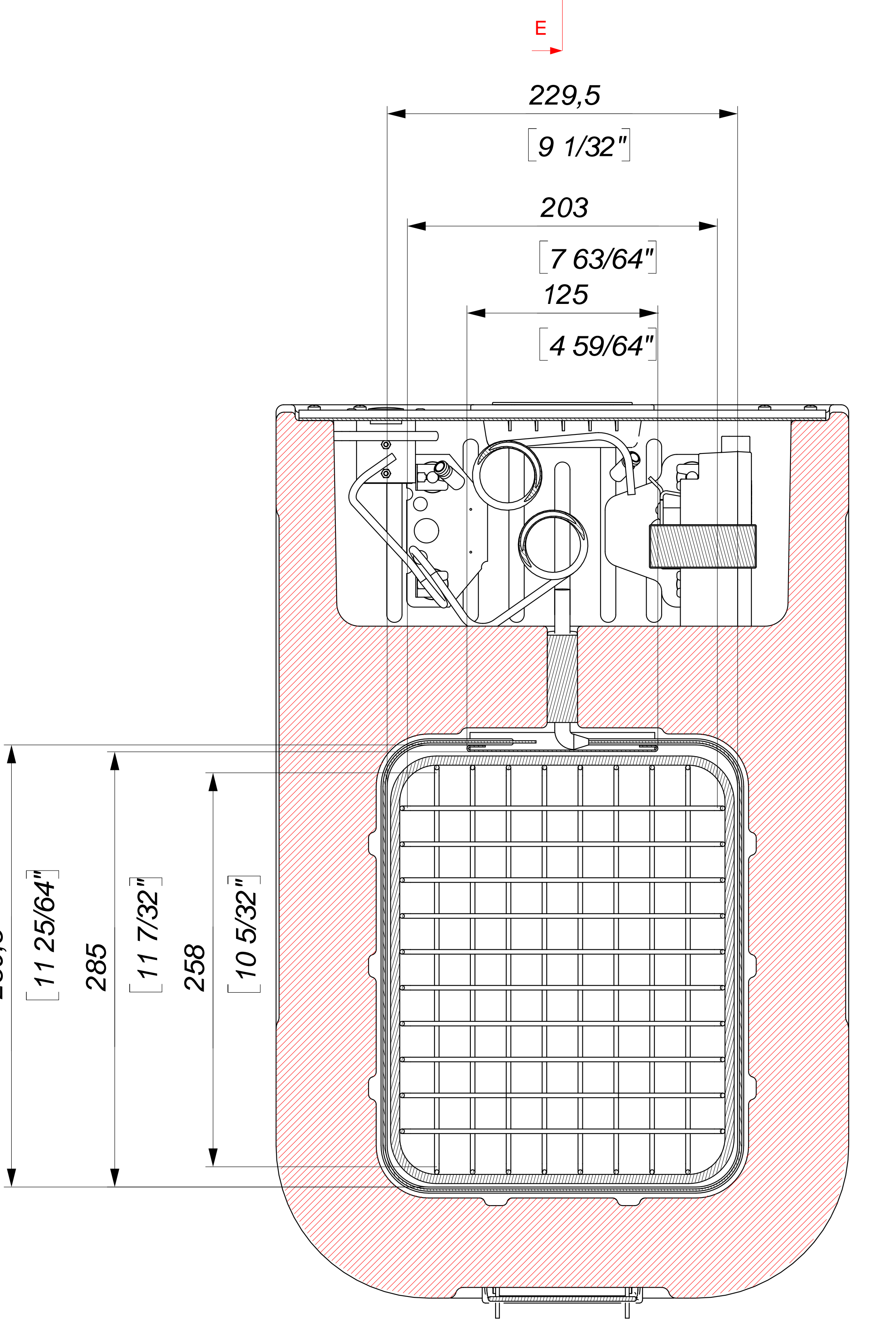
Sezione F-F SCALE 1 : 2
